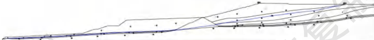
图 5.1-4 448.5m 滩顶标高坝体正常工况浸润线图
