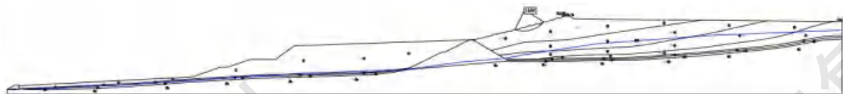
图5.1-10 现状滩顶标高443.95m（未运行状态）正常运行工况下坝体稳定性复核结果
