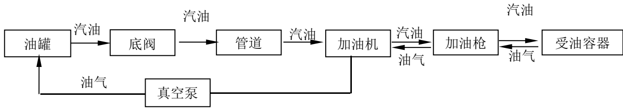
图 2.7-3 乙醇汽油加油工艺流程简图
