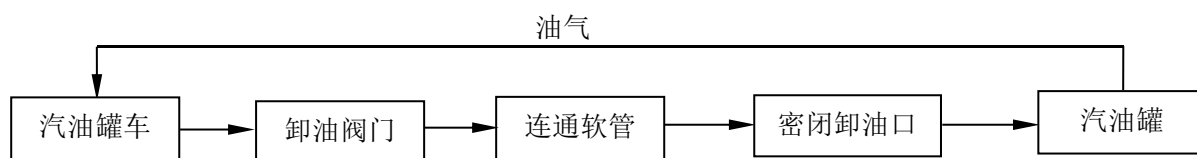
图 2.7-1 乙醇汽油罐车卸油工艺流程简图
