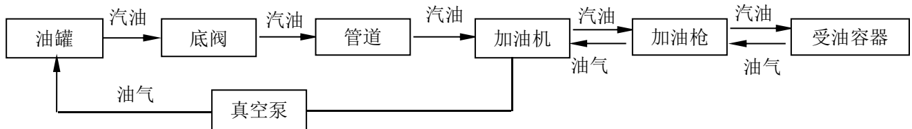
图 2.7-3 乙醇汽油加油工艺流程简图
