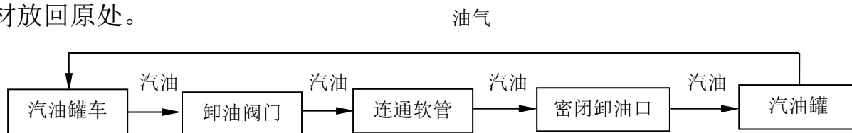
图 2.7-1 乙醇汽油罐车卸油工艺流程简图
