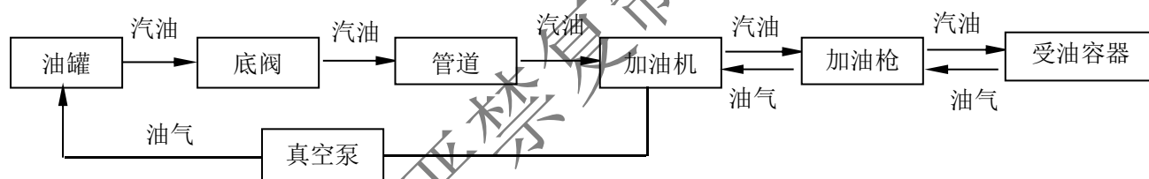
图 2.7-3 乙醇汽油加油工艺流程简图
