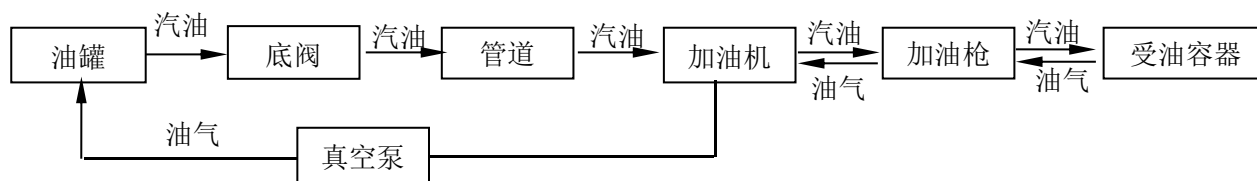
图 2.7-4 乙醇汽油加油工艺流程简图
