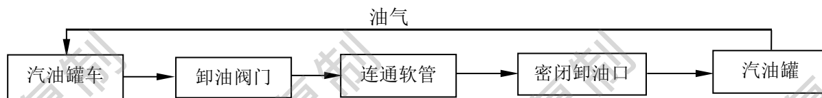
图 2.7-1 乙醇汽油罐车卸油工艺流程简图
