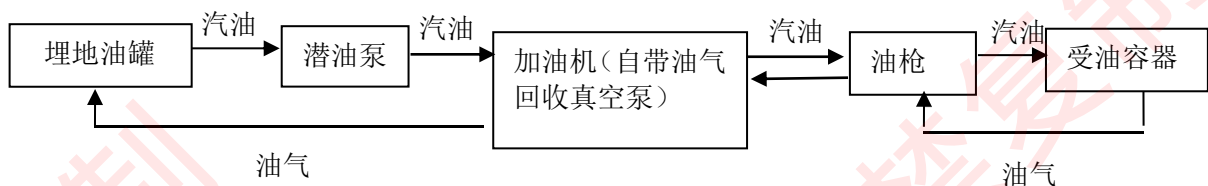
图 2.7.2-2 乙醇汽油加油工艺流程简图
