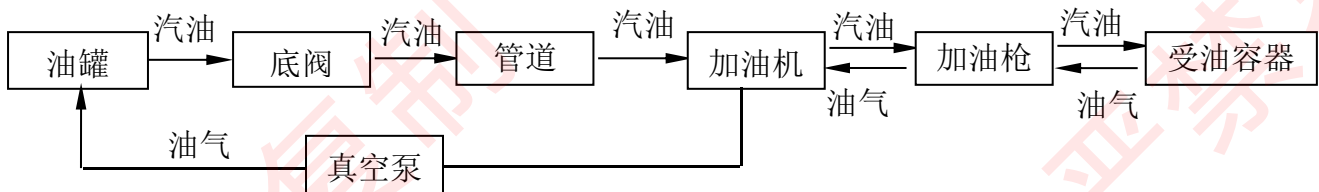
图 2.7.2-1 乙醇汽油加油工艺流程简图
