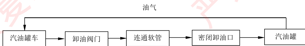
图 2.7.1-1 乙醇汽油罐车卸油工艺流程简图
