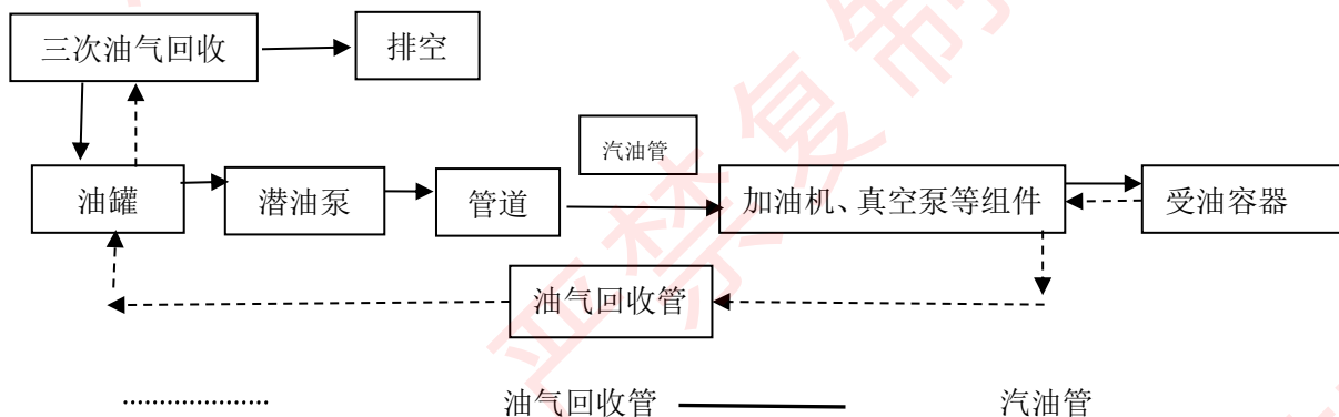
2.6.1 加油工艺流程框图
