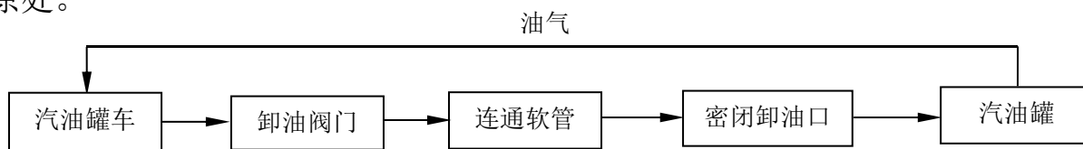
图 2.7-1 乙醇汽油罐车卸油工艺流程简图
