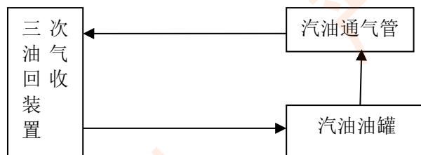
图 2.7-5 三次油气回收工艺流程简图
