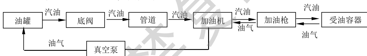
图 2.7-3 乙醇汽油加油工艺流程简图
