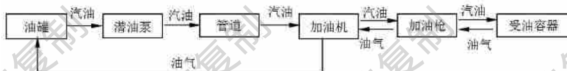
图 2.7-3 汽油加油工艺流程简图
