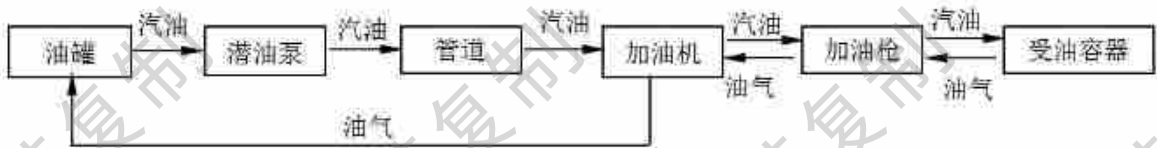
图 2.7-4 汽油加油工艺流程简图
