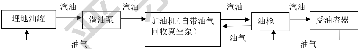
图 2.7-4 乙醇汽油潜油泵式加油工艺流程简图
