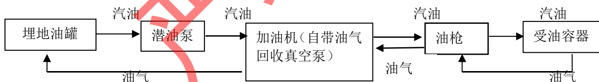
图 2.7-4 乙醇汽油加油工艺流程简图
