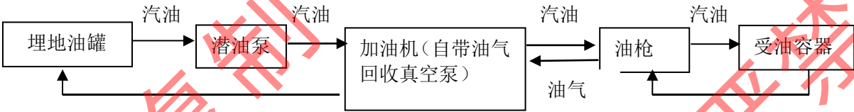
图 2.7-3 乙醇汽油加油工艺流程简图
