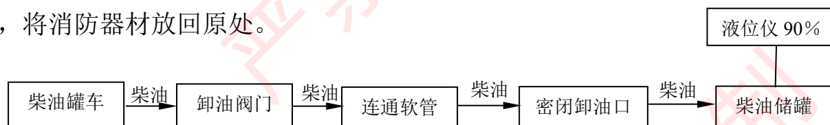
图 2.7-2 柴油罐车卸油工艺流程简图
