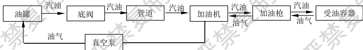
图 2.7-3 乙醇汽油加油工艺流程简图
