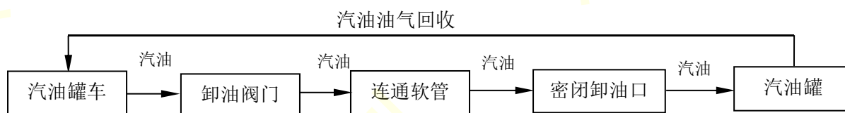
图 2.7-1 乙醇汽油罐车卸油工艺流程简图
