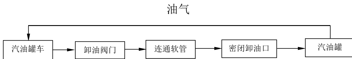
图 2.7-1 乙醇汽油罐车卸油工艺流程简图
