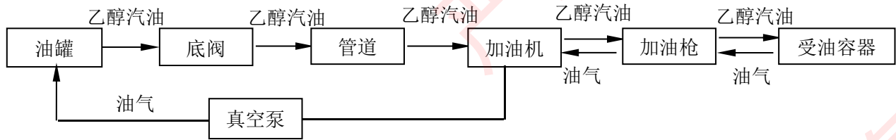
图 2.7-3 乙醇汽油加油工艺流程简图
