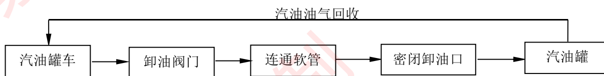
图 2.7-1 汽油罐车卸油工艺流程简图
