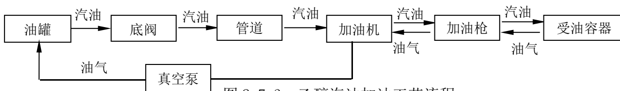
图 2.7-3 乙醇汽油加油工艺流程
