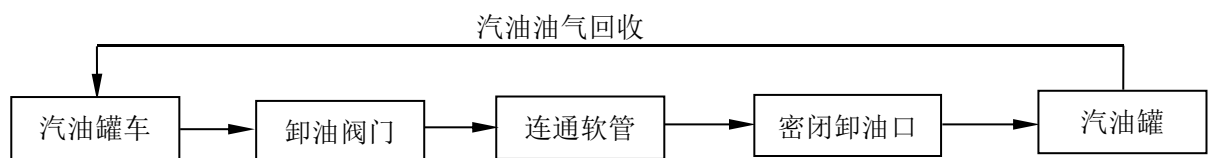
图 2.7-1 汽油罐车卸油工艺流程简图
