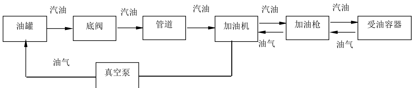
图 2.7-3 汽油加油工艺流程简图
