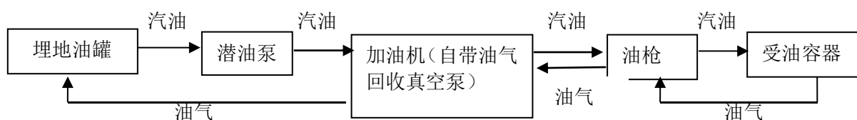
图 2.7-4 乙醇汽油潜油泵式加油工艺流程简图
