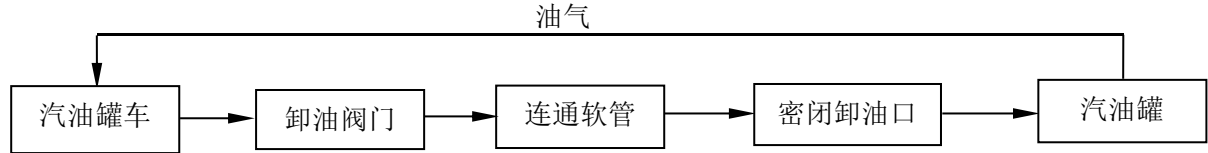
图 2.7-1 乙醇汽油罐车卸油工艺流程简图
